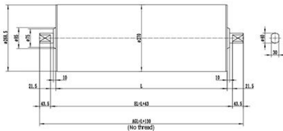
TM270H Idler roller
