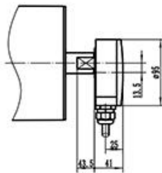
TM270H Idler roller
